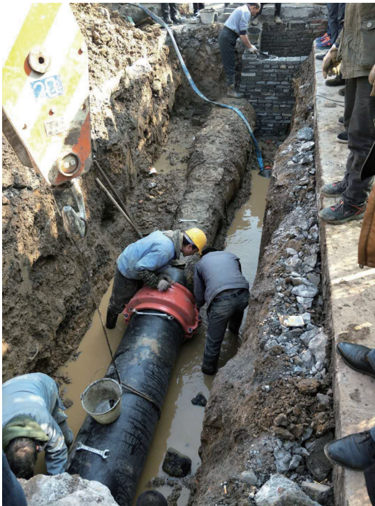
▲安装现场
