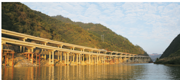
▲吊装运输最后一 片T梁
